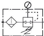
Zweifachblock (Filter und Regler)
