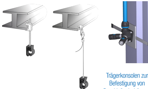
Hängende Montage
