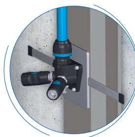
ANBRINGUNG AN IPN-/HEA-TRÄGER MIT TRÄGERKONSOLE
